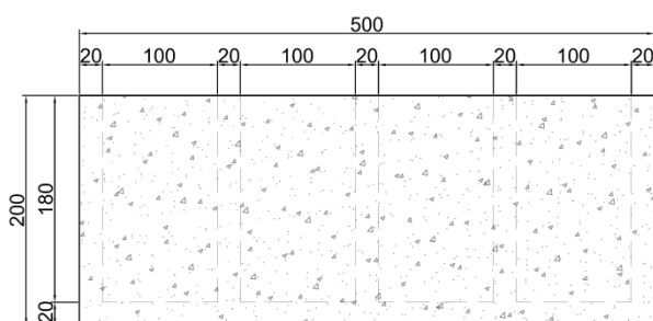
PROSPETTO
