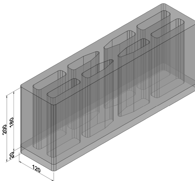
VISTA ASSONOMETRICA
